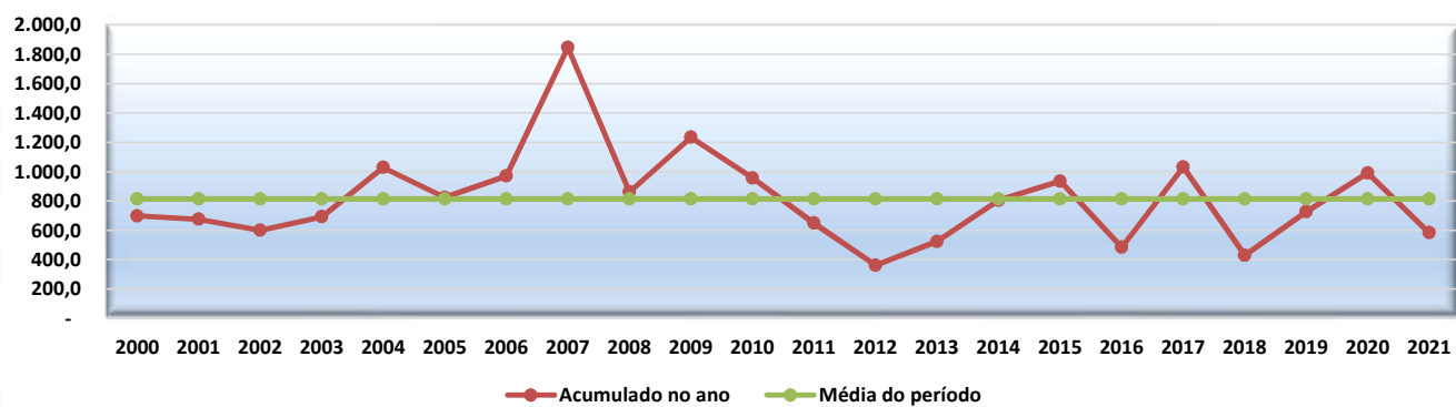
Município de Ribeirópolis Gráfico 03 - Pluviosidade Acumulada Anual e Média do Período - 2000 a 2021
