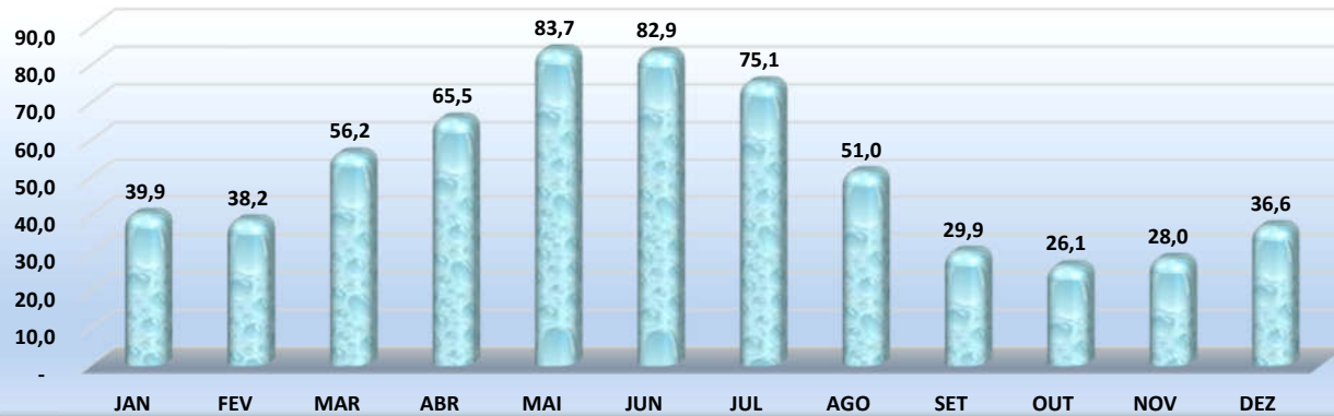
Município de Poço Verde Gráfico 01 - Pluviosidade Média Mensal - 2000 a 2021
