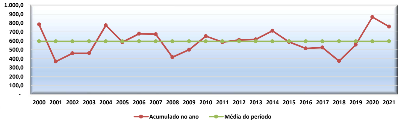
Município de Poço Verde Gráfico 03 - Pluviosidade Acumulada Anual e Média do Período - 2000 a 2021
