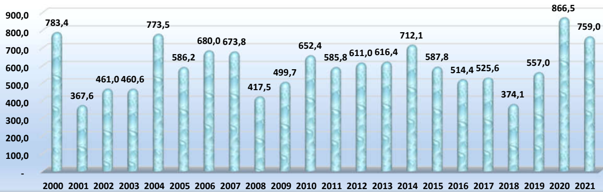
Município de Poço Verde Gráfico 02 - Pluviosidade Média Acumulada Anual - 2000 a 2021
