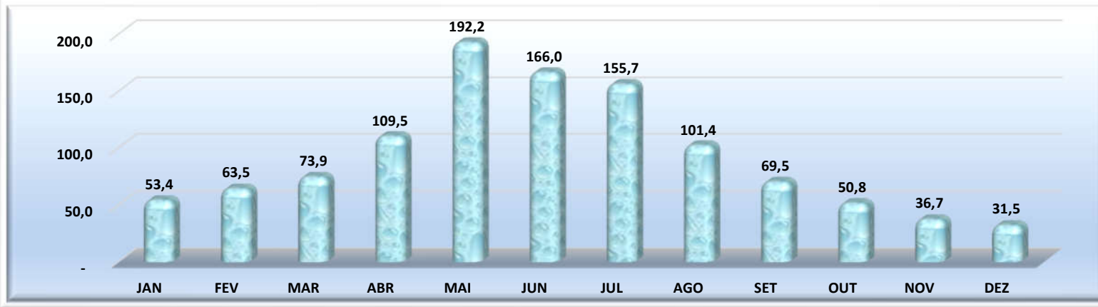
Município de Lagarto Gráfico 01 - Pluviosidade Média Mensal - 2000 a 2021
