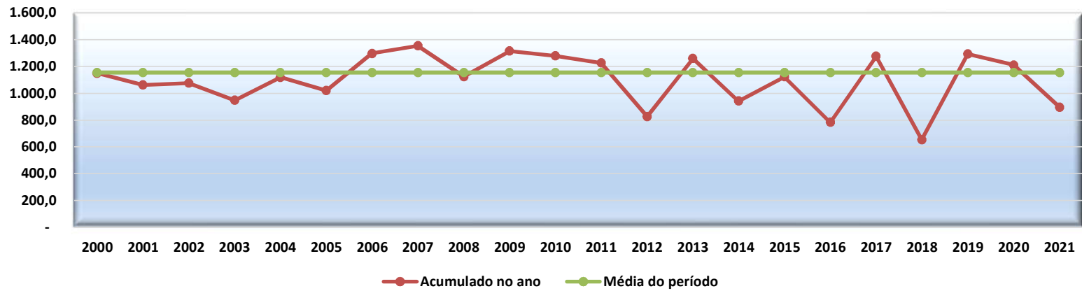
Município de Lagarto Gráfico 03 - Pluviosidade Acumulada Anual e Média do Período - 2000 a 2021
