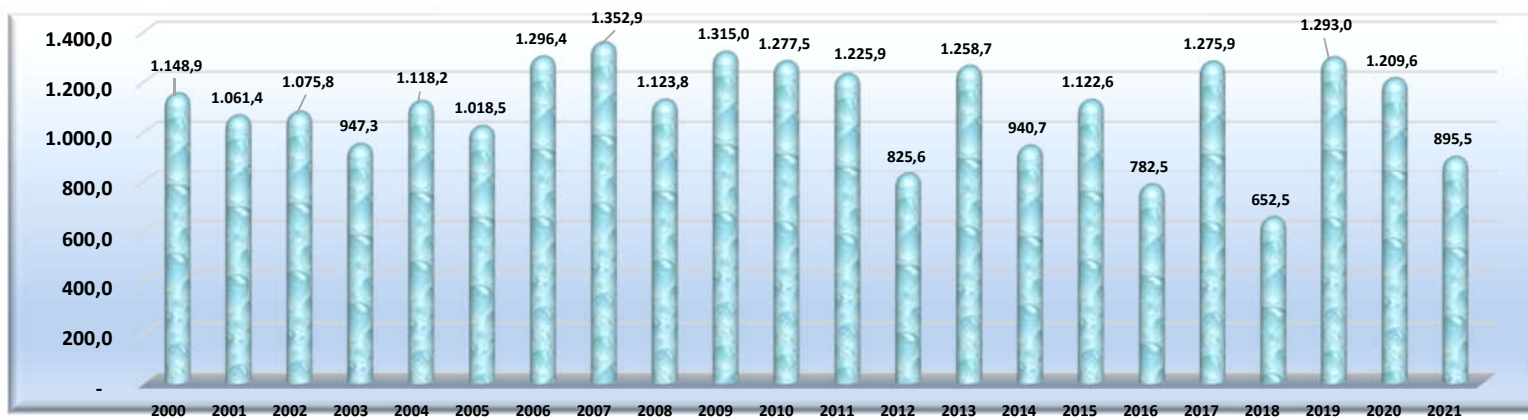
Município de Lagarto Gráfico 02 - Pluviosidade Média Acumulada Anual - 2000 a 2021
