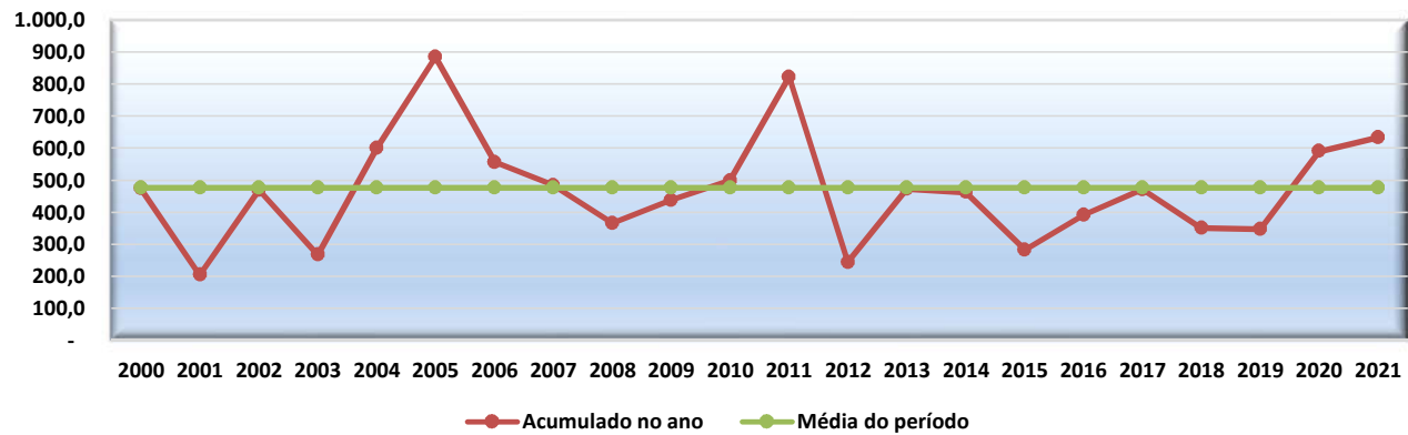
Município de Canindé do São Francisco Gráfico 03 - Pluviosidade Acumulada Anual e Média do Período - 2000 a 2021
