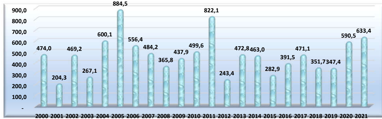
Município de Canindé do São Francisco Gráfico 02 - Pluviosidade Média Acumulada Anual - 2000 a 2021
